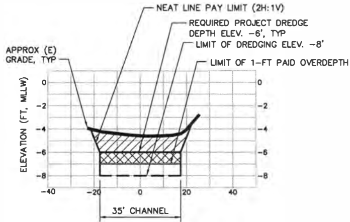
DREDGE UNIT 5 (FINGER 3) STA 1+25
