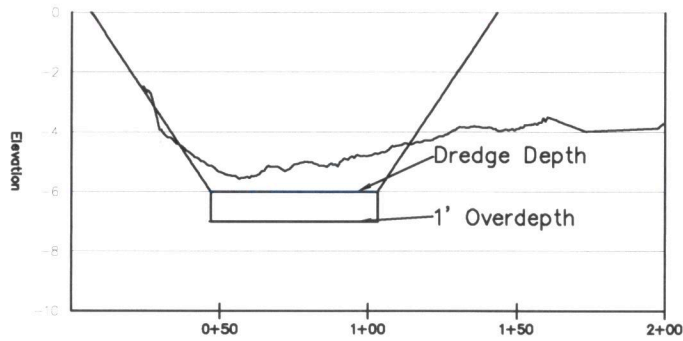
Section 2 Horizontal Scale: 1" = 20' Vertical Scale: 1" = 5'
