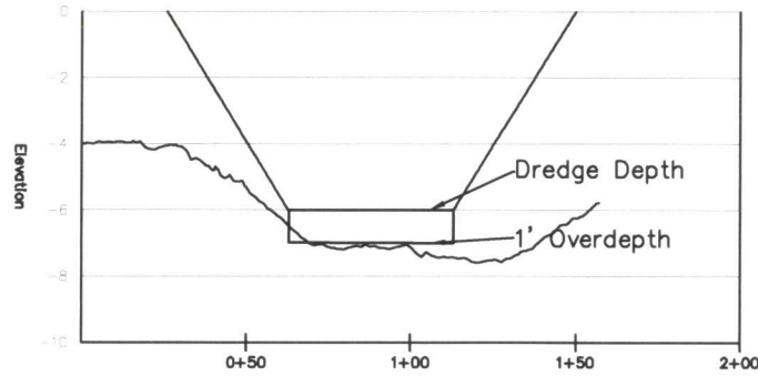
Section 1 Horizontal Scale: 1" = 20' Vertical Scale: 1" = 5'
