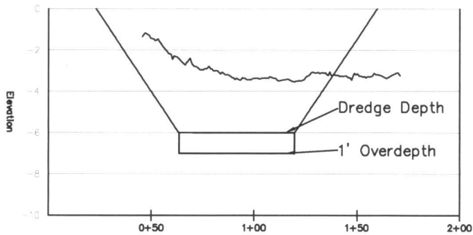
Section 3 Horizontal Scale: 1" = 20' Vertical Scale: 1" = 5'
